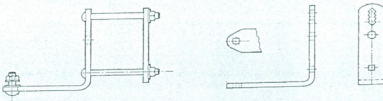
شکل ۲ - دستک نصب نوع «سی»
