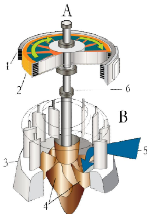
یک توربین آبی وصل شده به یک مولد الکتریکی.
