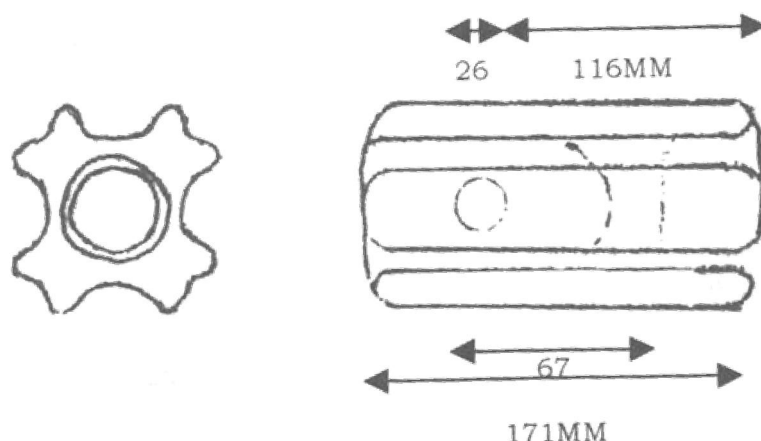
شکل ۱۴- مقره مهار
