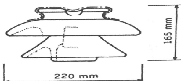
شکل ۶- ب - مقره سوزنی برای ولتاژ ۲۰ کیلو ولت ولتاژ جرعه سطح خشک آن ۱۱۰ کیلو ولت ولتاژ جرعه سطح مرطوب آن ۷۰ کیلو ولت
