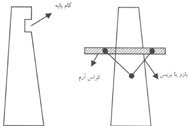
شکل ۱- گام در پایه های چوبی
